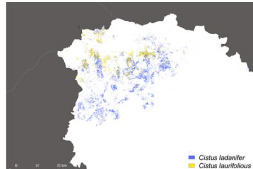
Clasificación de jarales mediante teledetección
